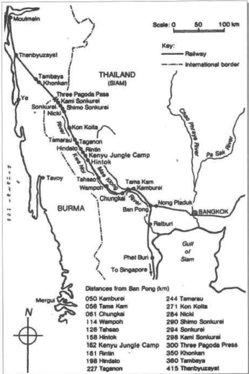
泰緬連接鐵道路線図（出所：豪州国立文書館サイト）
